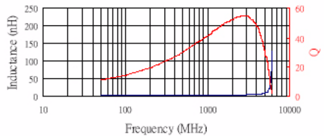
AL03BT5N6
