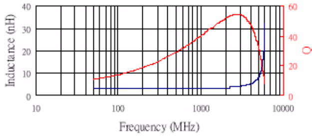
AL03BT4N7
