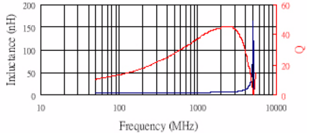
AL03BT8N2
