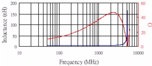
AL03BT6N8
