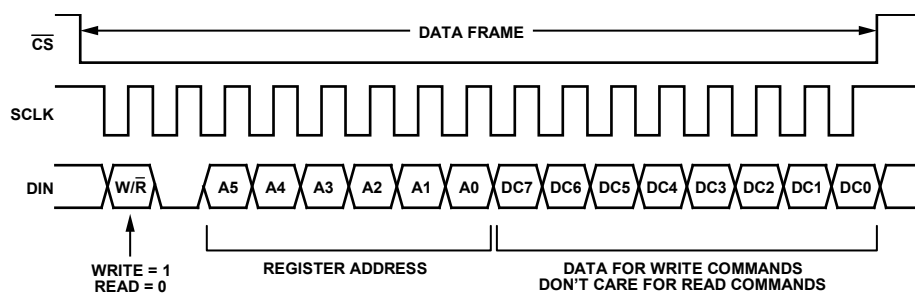
Figure 27. DIN Bit Sequence
