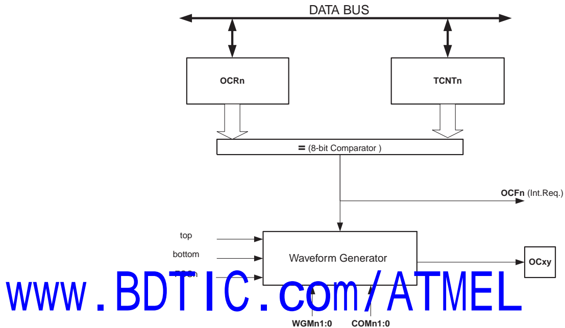
Figure 55. 输出比较单元方框图
