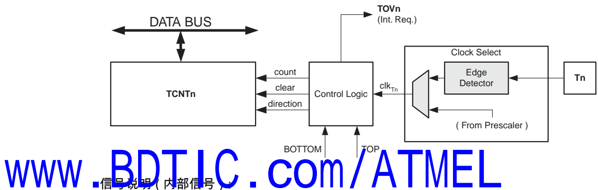
Figure 28. 计数器单元方框图
