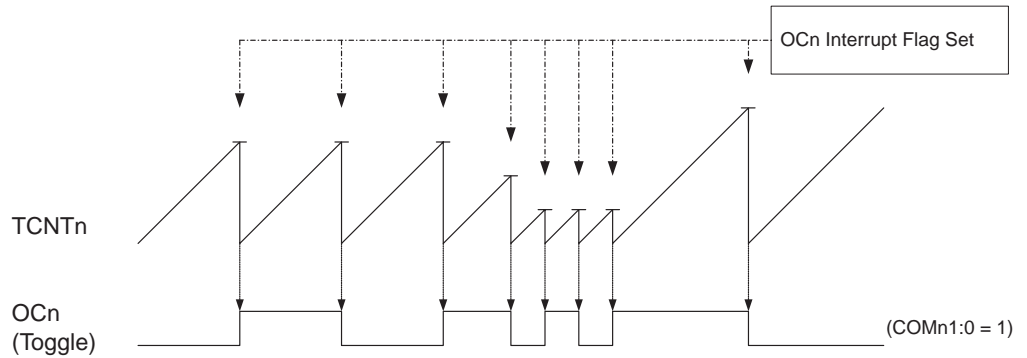
Figure 31. CTC 模式的时序图
