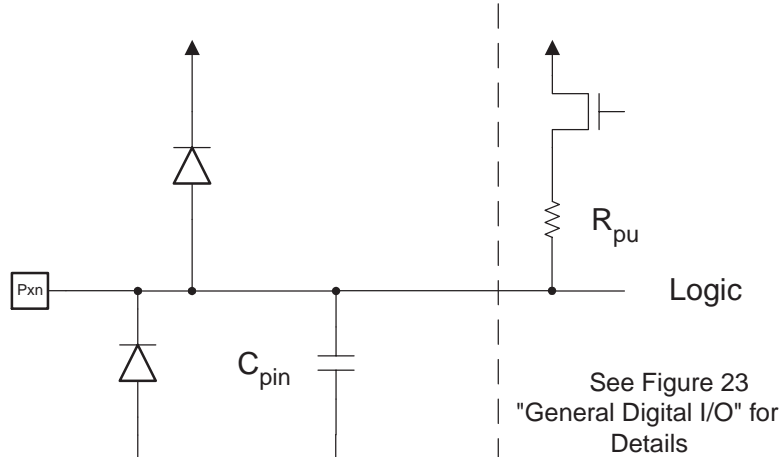
Figure 22. I/O 引脚等效原理图
