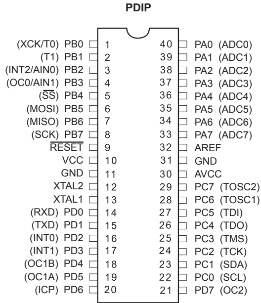
Figure 1. ATmega32 的引脚
