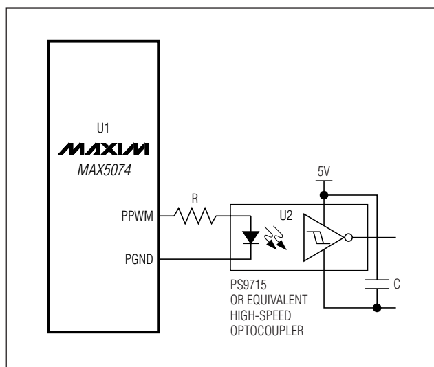
图 2. 利用高速光耦驱动二次侧同步整流器
