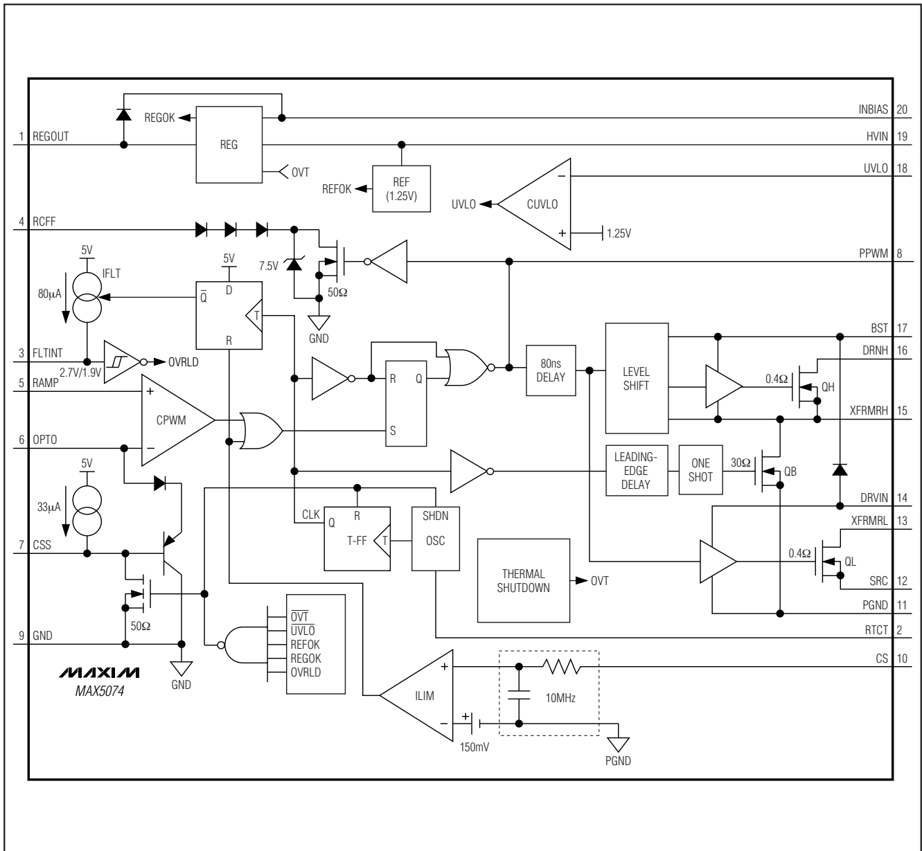
图 1. 内部框图
