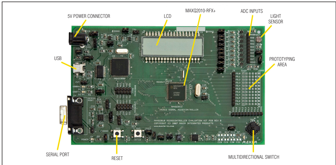
图1. MAXQ2010评估板
