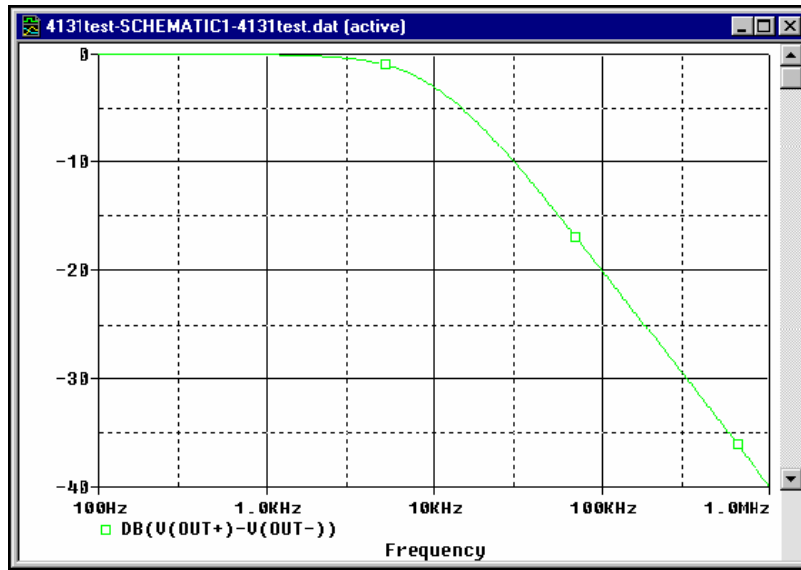
图 21. 仿真结果
