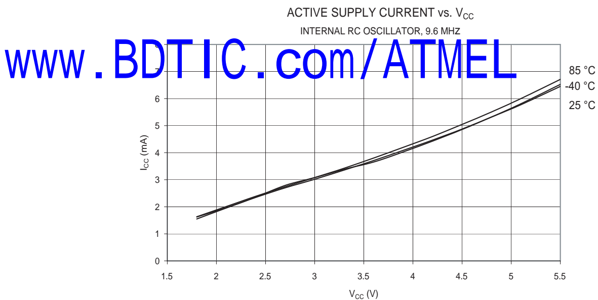
Figure 65. 工作电流和 V_{CC} 的关系 (内部 RC 振荡器, 9.6MHz)
