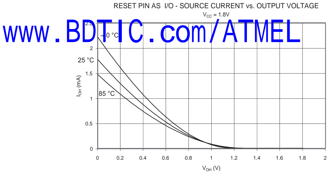
Figure 95. Reset 引脚作为 I/O – 源电流和输出电压的关系 ( V_{CC} = 1.8V )
