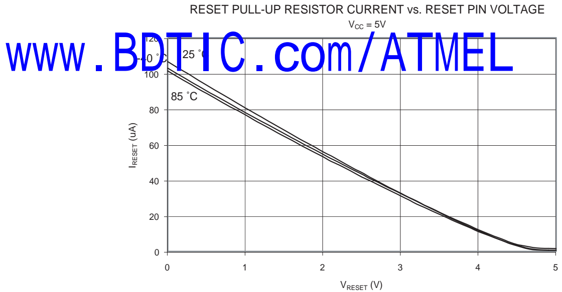
Figure 79. 复位 (Reset) 引脚上拉电阻电流和 Reset 引脚电压的关系 ( V_{CC} = 5V )
