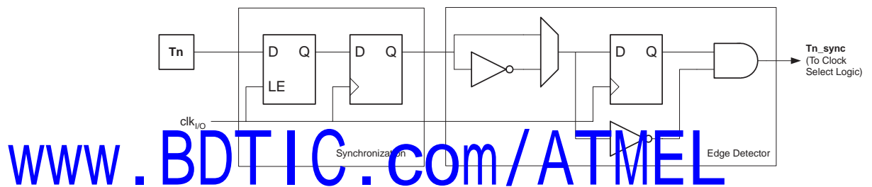
Figure 36. T0 引脚采样
