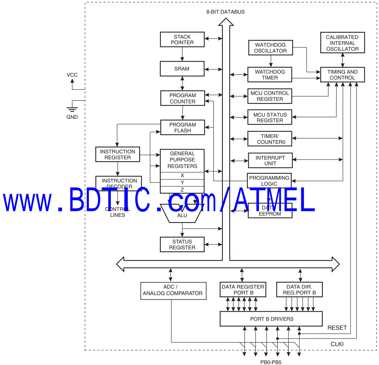
Figure 2. ATtiny13 结构框图
