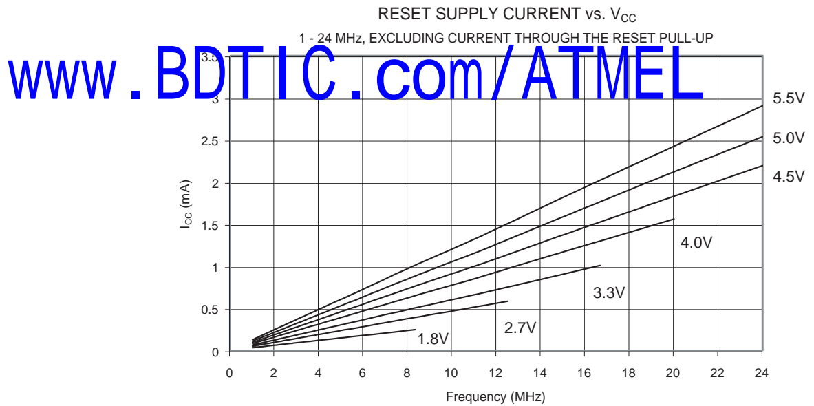
Figure 127. 复位电流和 V_{CC} 的关系 (1 - 24MHz, 包括流经复位上拉电阻的电流)
