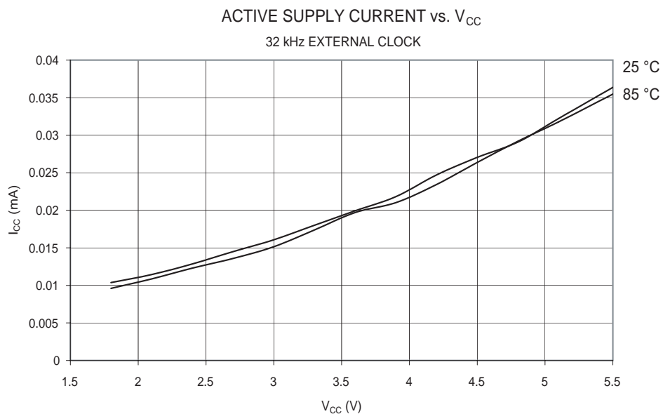
Figure 68. 工作电流和 V_{CC} 的关系 (32 kHz 外部时钟)
