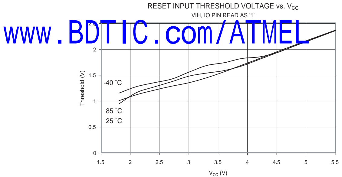
Figure 105. Reset 输入门限电压和 V_{CC} 的关系 ( V_{IH} , Reset 引脚读值为 '1')
