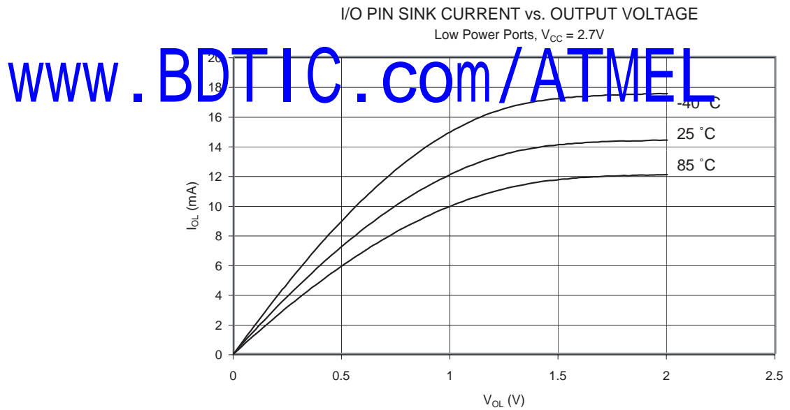
Figure 85. I/O 引脚吸收电流和输出电压的关系 (低功端口, V_{CC} = 2.7V )
