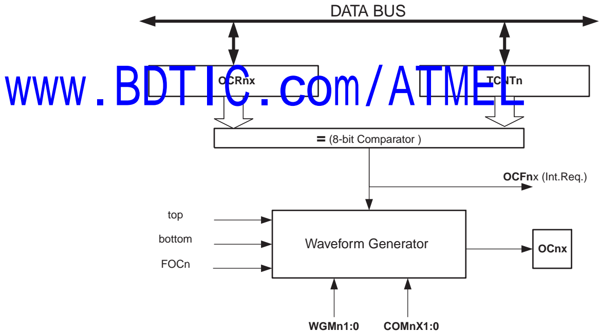
Figure 27. 输出比较单元方框图
