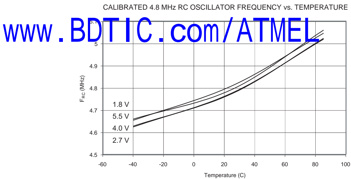
Figure 117. 标定 4.8 MHz RC 振荡器频率与温度的关系
