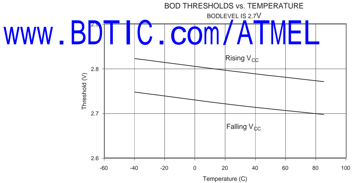
Figure 109. BOD 门限值和温度的关系 (BOD 电平为 2.7V)
