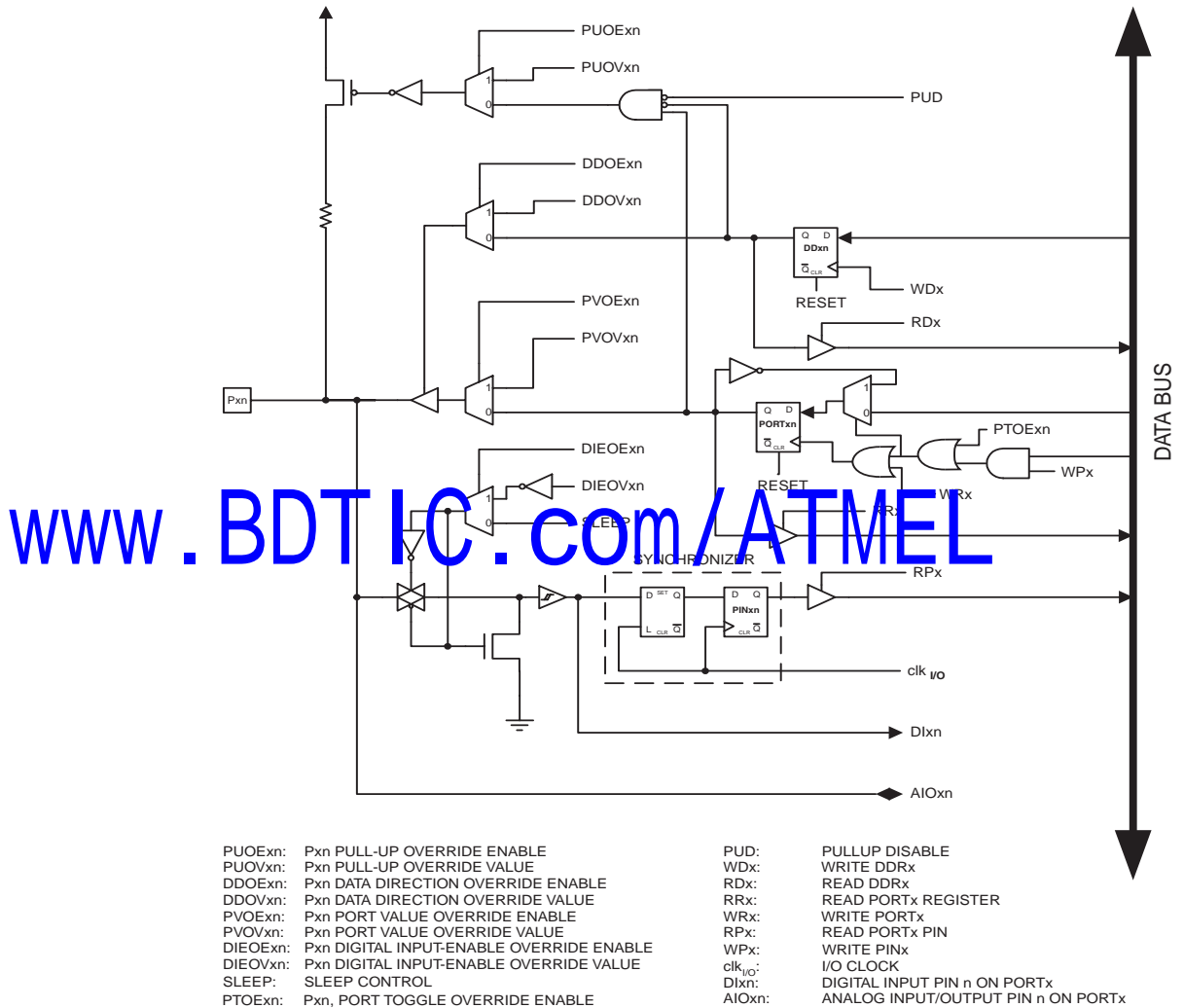
Figure 24. 端口的第二功能 (1)
