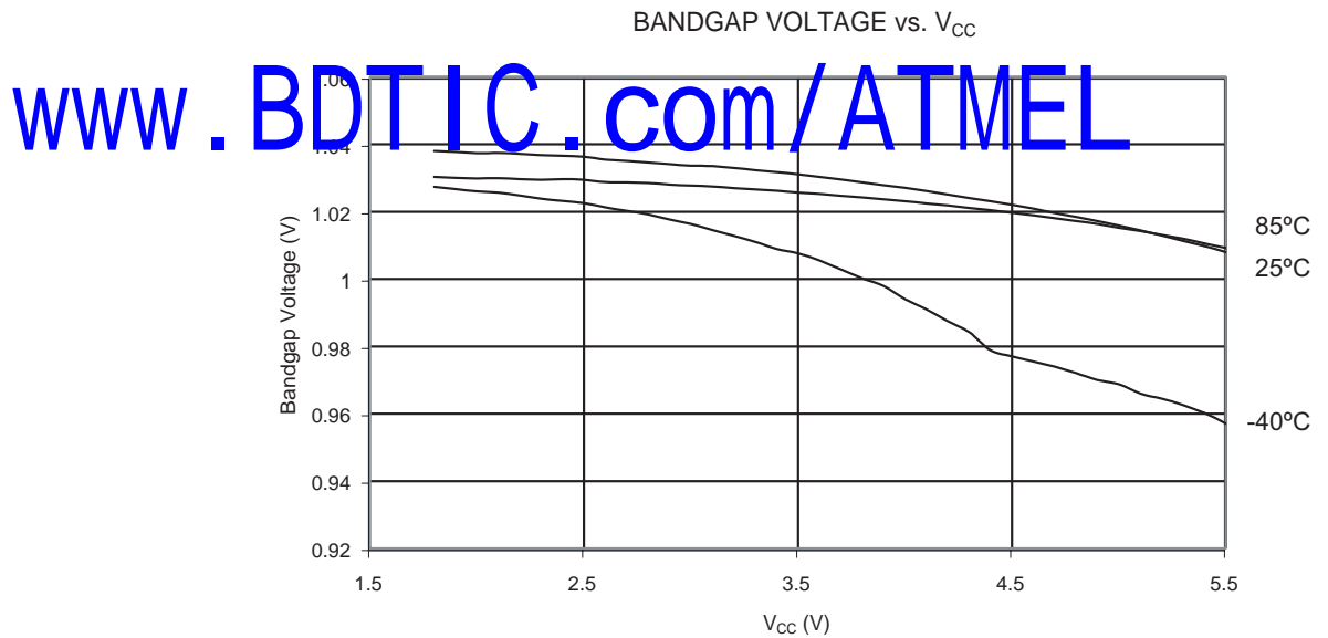
Figure 111. 能隙电压和 V_{CC} 的关系
