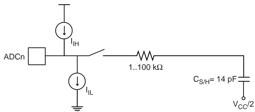
Figure 46. 模拟输入电路
