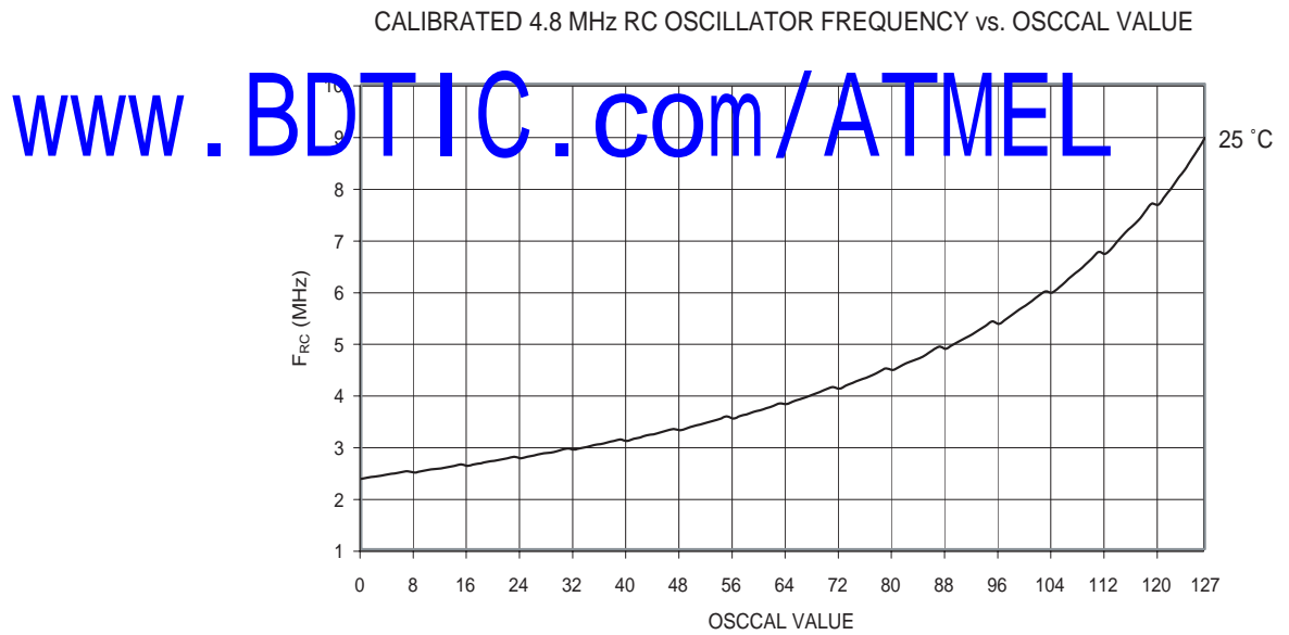
Figure 119. 标定 4.8 MHz RC 振荡器频率与 OscCal 值的关系
