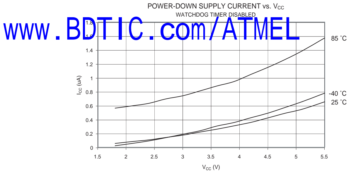
Figure 75. 掉电模式电流和 V_{CC} 的关系 (看门狗定时器禁用)
