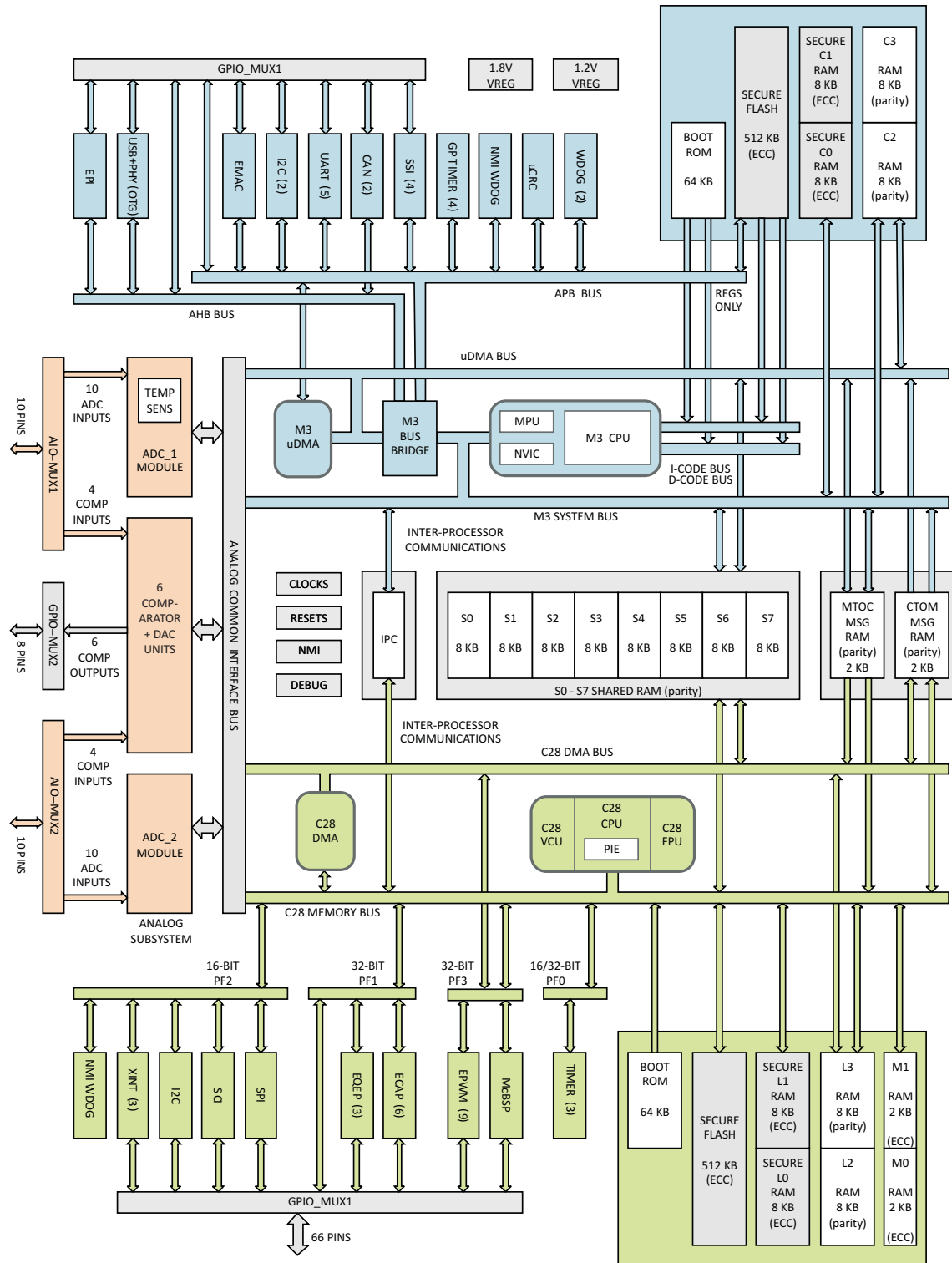
图 1-1. 功能方框图
