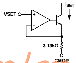
Figure 28. VSET Interface
