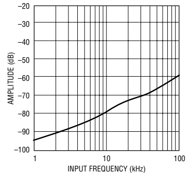
总谐波失真与输入频率的关系曲线
