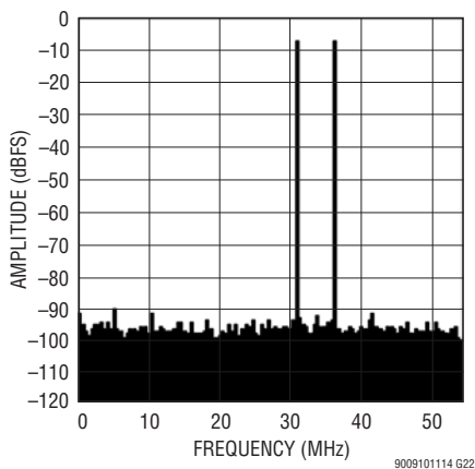
LTM9010-14: 8k Point 2-Tone FFT, f_{IN} = 70\text{MHz} , 75\text{MHz} , -7\text{dBFS} per Tone, 105\text{Mpsps}
