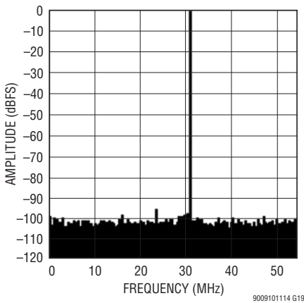
LTM9010-14: 8k Point FFT, f_{IN} = 30\text{MHz} , -1\text{dBFS} , 105\text{Mpsps}
