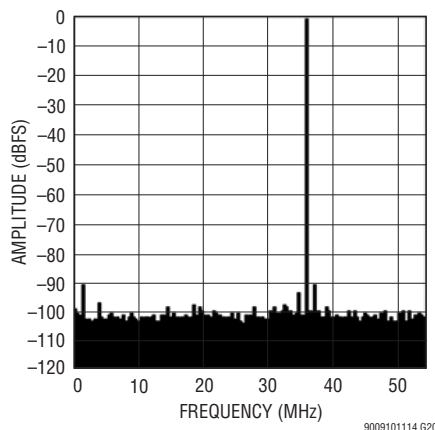
LTM9010-14: 8k Point FFT, f_{IN} = 70\text{MHz} , -1\text{dBFS} , 105\text{Mpsps}
