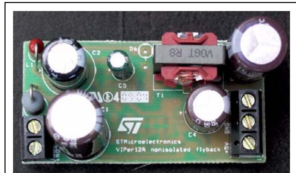
STEVAL-ISA006V1
