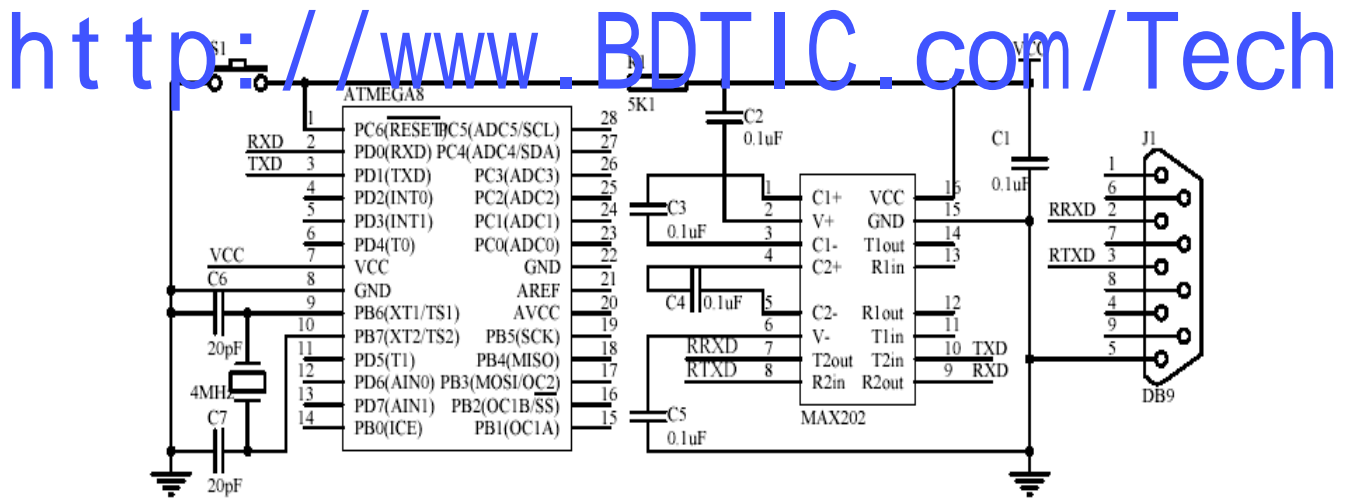
图 4-1 UART 实现 I/O 流电路原理图
