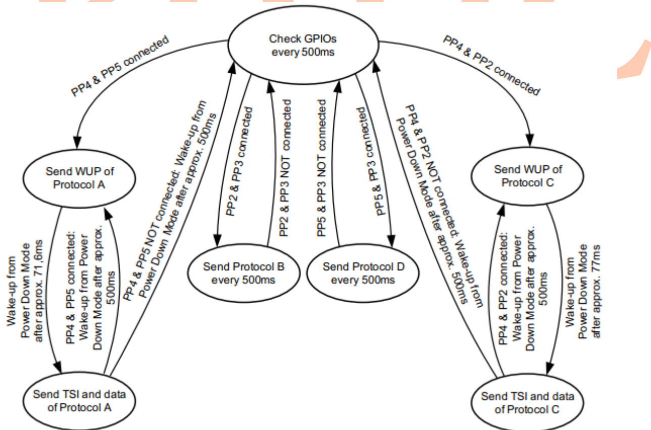
图 1 PMA71xx/PMA51xx 射频协议示例软件实现的状态图
