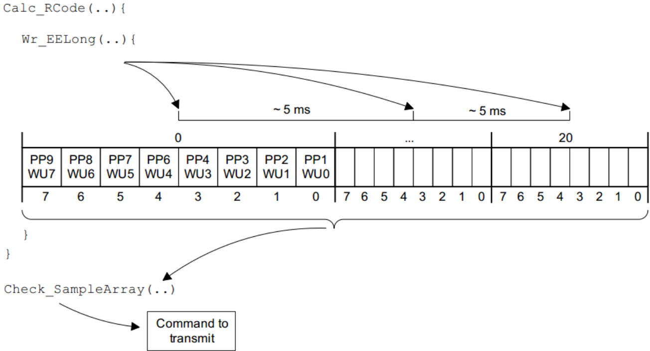
图 4 模拟 EEPROM 写访问期间的端口采样
