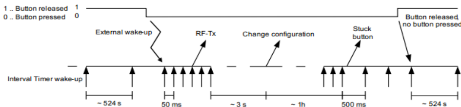
图 3 按钮按下和间隔定时器的时间设置
