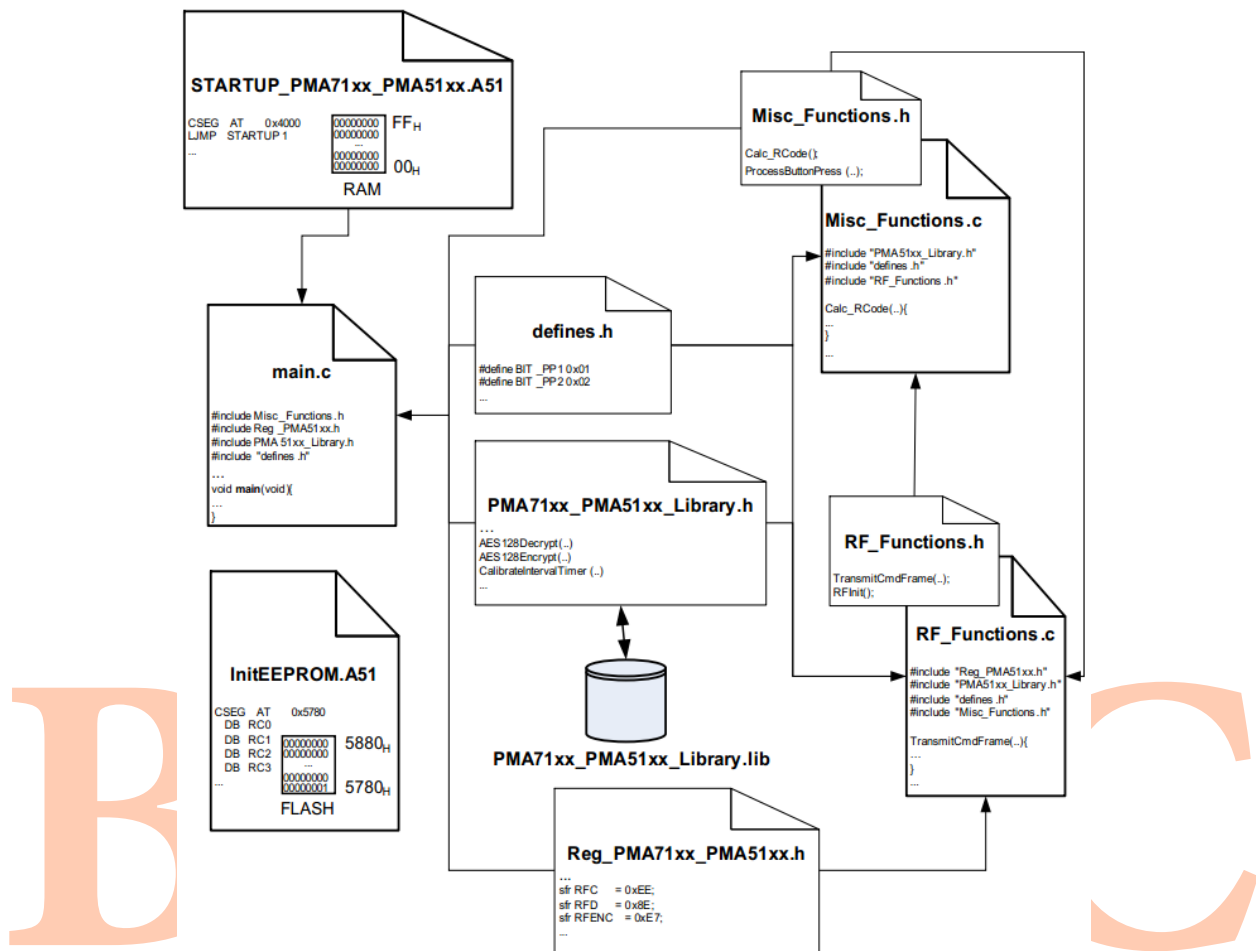
图1 PMAfob 软件示例的文件结构
