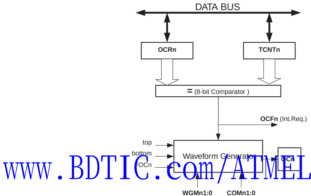
Figure 29. 输出比较单元方框图
