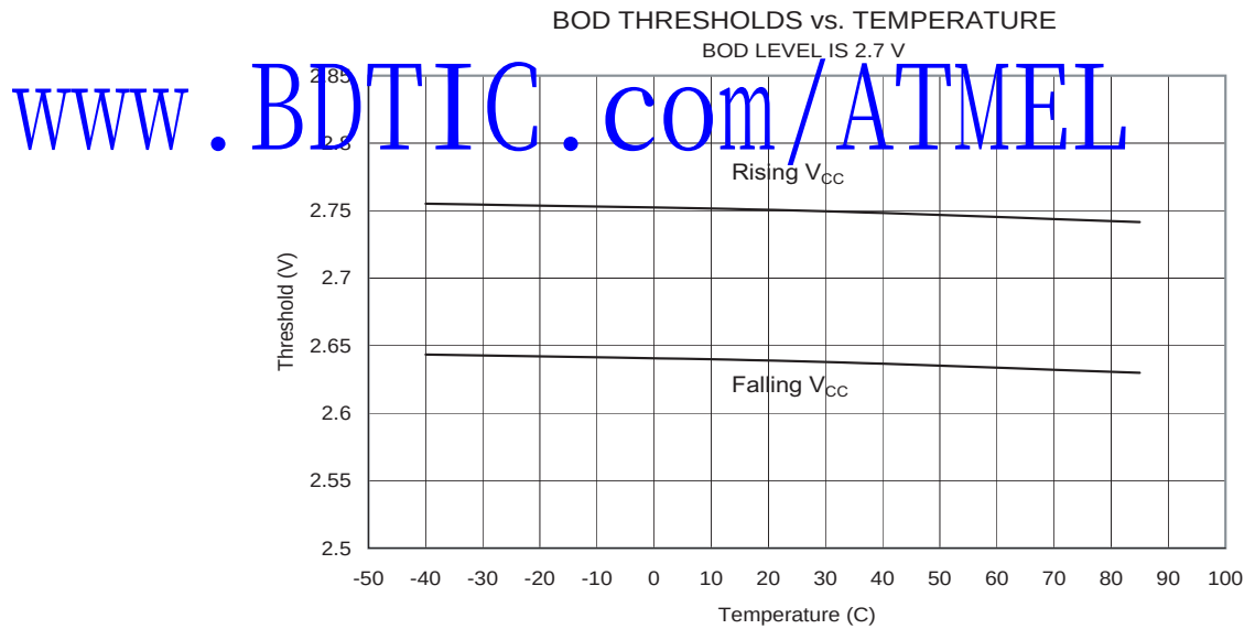
Figure 170. BOD 门限值和温度的关系 (BOD 电平为 2.7V)
