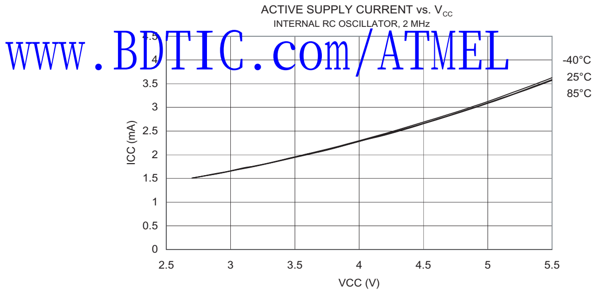
Figure 134. 工作电流和 V_{CC} 的关系 (内部 RC 振荡器, 2 MHz)
