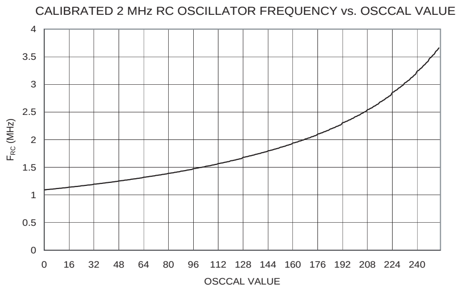
Figure 183. 校准的 2 MHz RC 振荡器频率和 Oscal 数值的关系
