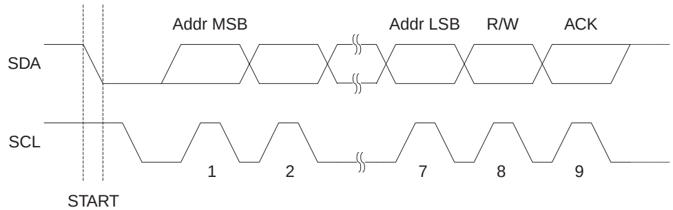
Figure 79. 地址包格式
