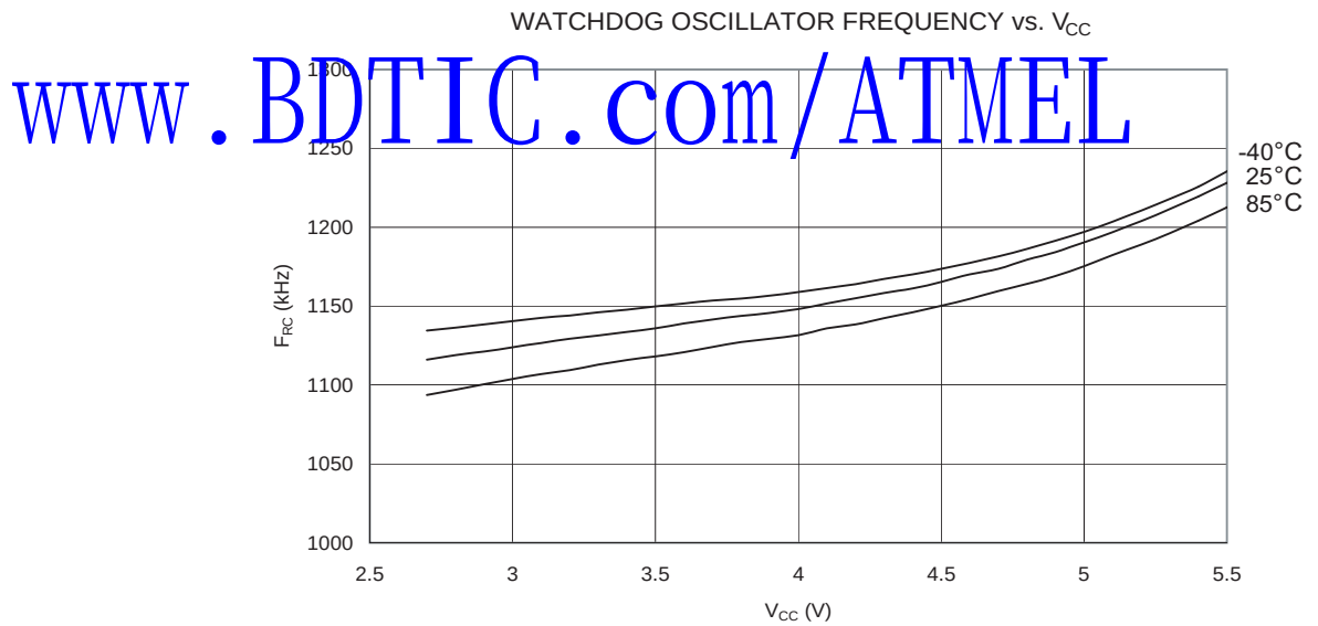
Figure 174. 看门狗振荡器频率和 V_{CC} 的关系
