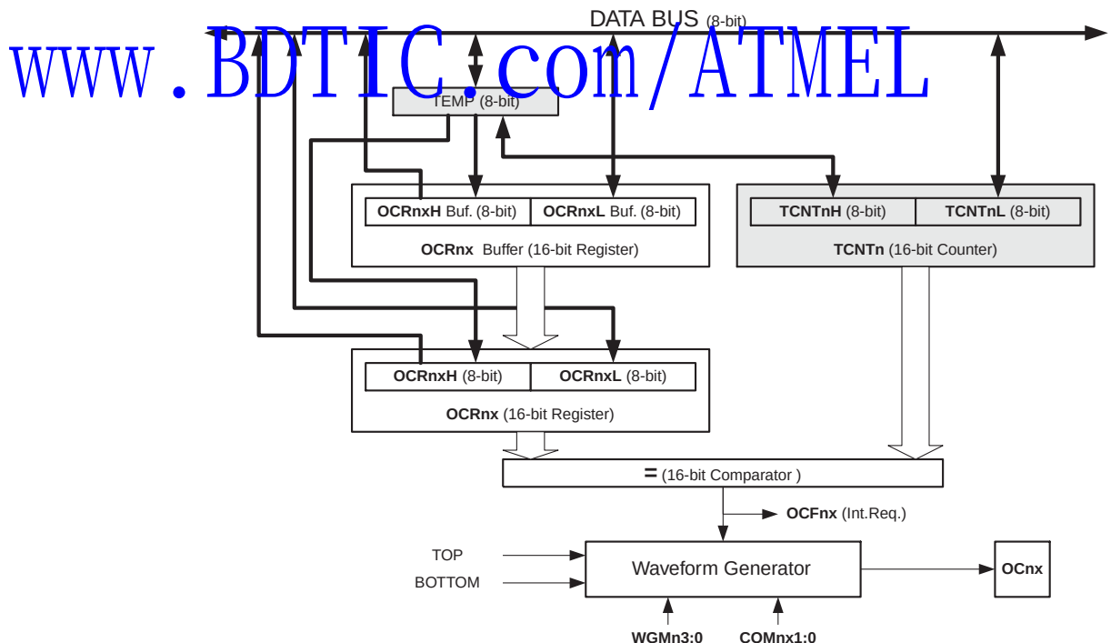
Figure 43. 输出比较单元方框图
