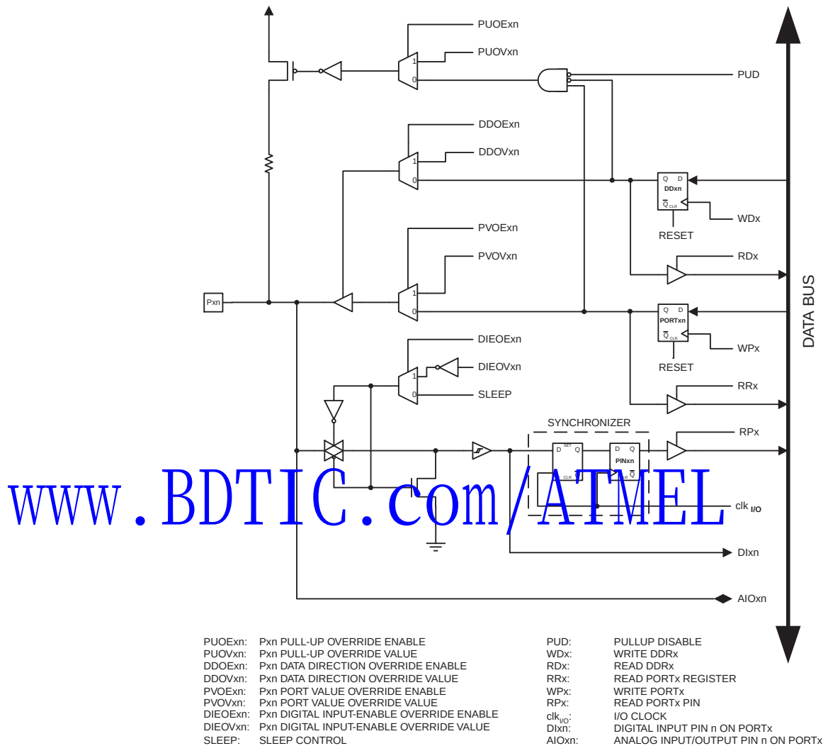
Figure 26. 端口的第二功能 (1)
