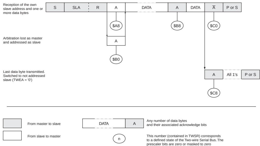
Figure 93. 从机发送模式的格式和状态
