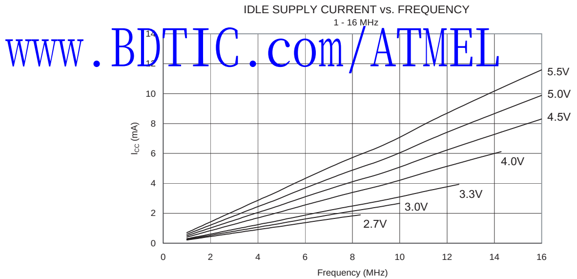
Figure 138. 空闲模式电流和工作频率 (1 - 16 MHz) 的关系
