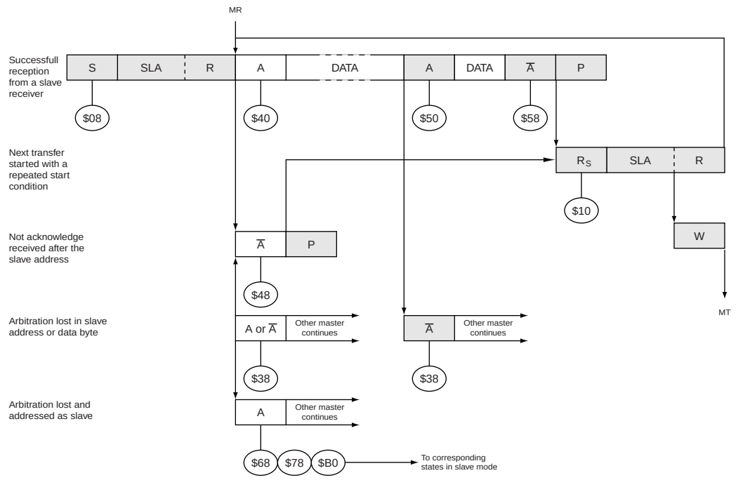
Figure 89. 主机接收模式的格式和状态
