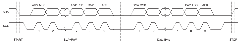
Figure 81. 典型的数据传送
