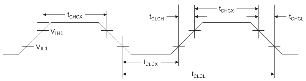
Figure 126. 外部时钟驱动波形
