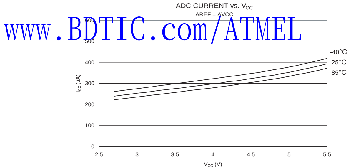
Figure 188. ADC 电流和 V_{CC} 的关系 (AREF = AVCC)
