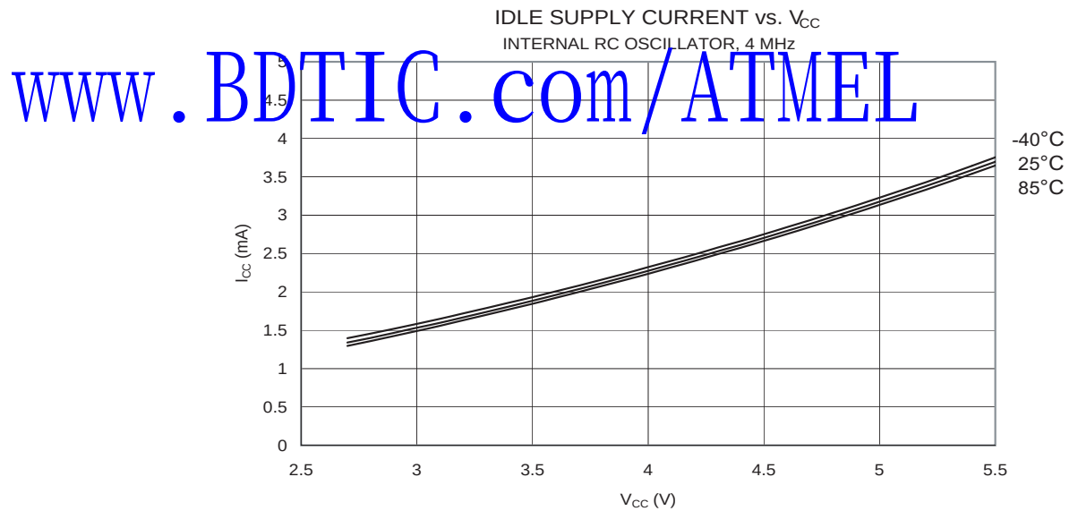
Figure 140. 空闲模式电流和 V_{CC} 的关系 (内部 RC 振荡器, 4 MHz)
