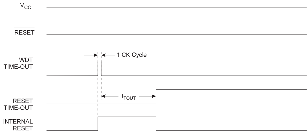
Figure 20. 工作过程中发生看门狗复位
