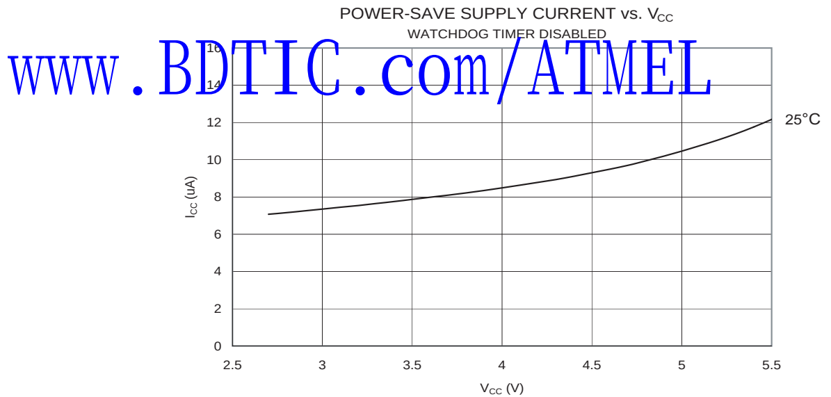
Figure 146. 省电模式电流和 V_{CC} 的关系 (看门狗定时器禁用)
