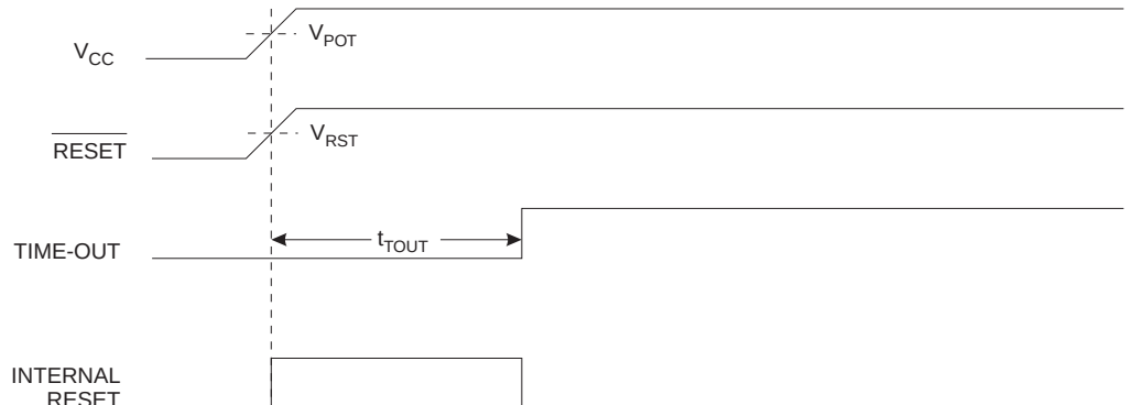
Figure 16. MCU 启动过程, RESET 连接到 V_{CC}
