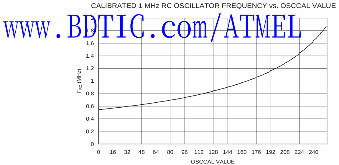
Figure 186. 校准的 1 MHz RC 振荡器频率和 Oscal 数值的关系
