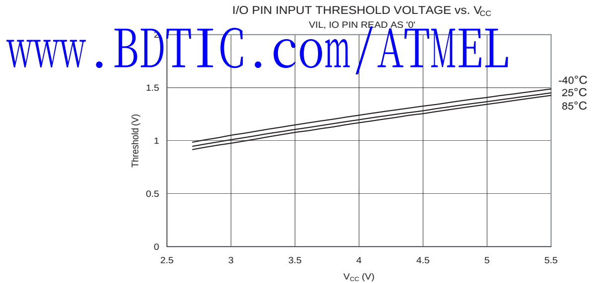
Figure 164. I/O 引脚输入门限电压和 V_{CC} 的关系 ( V_{IL} , I/O 引脚读值为 '0')
