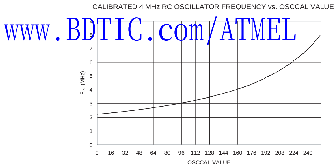
Figure 180. 校准的 4 MHz RC 振荡器频率和 Oscal 数值的关系
