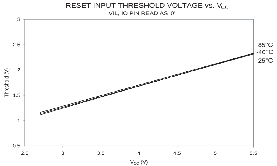
Figure 167. Reset 输入门限电压和 V_{CC} 的关系 ( V_{IL} , Reset 引脚读出值为 '0')
