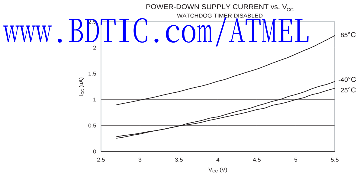
Figure 144. 掉电模式电流和 V_{CC} 的关系 (看门狗定时器禁用)
