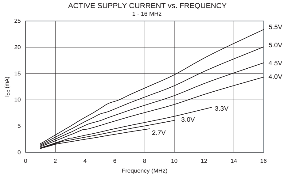
Figure 131. 工作电流和工作频率 (1 - 16 MHz) 的关系
