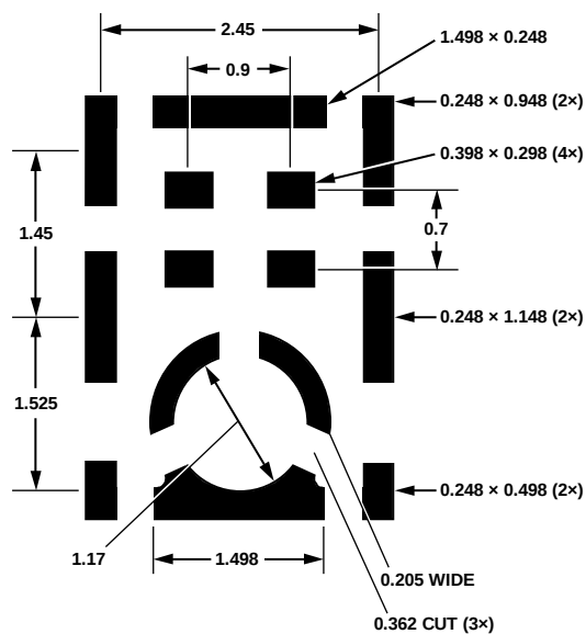
图9. 建议焊膏模板图形布局
