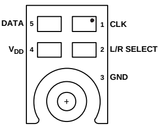
图4. 引脚配置(底视图)
