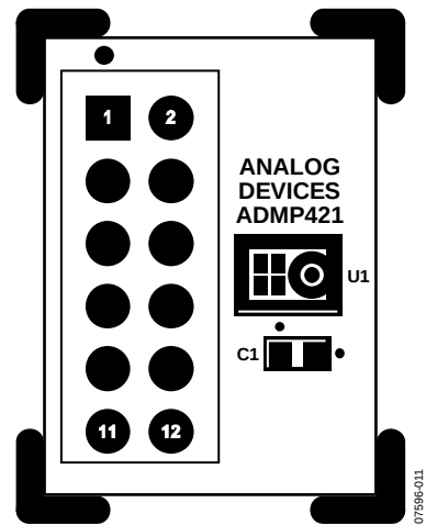
图11. ADMP421评估板布局图
