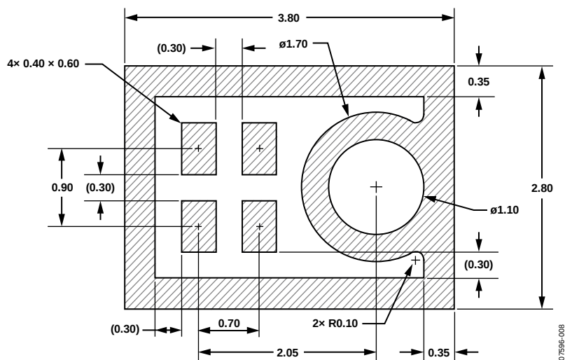
图8. 建议PCB焊盘图形布局
